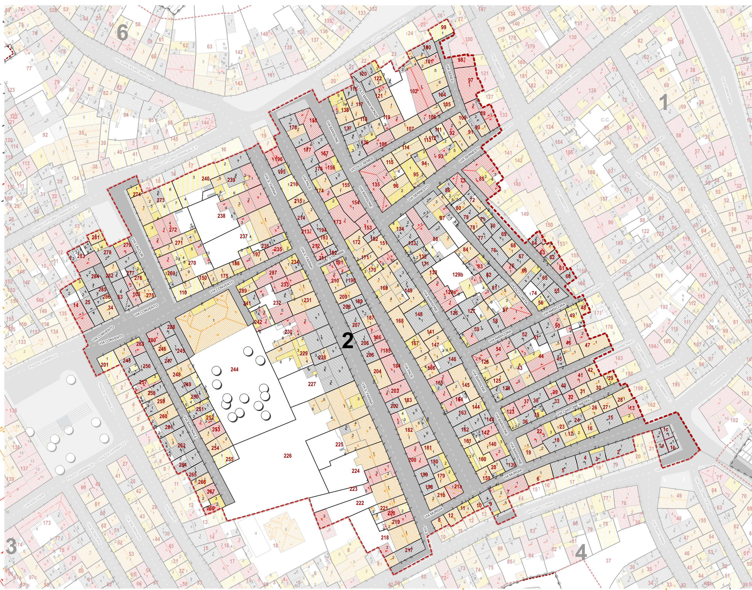
Planimetria delle coperture di stato attuale scale 1:1000
