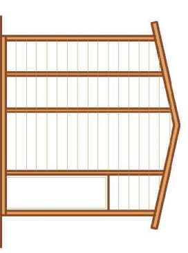
PROSPETTO LATERALE
