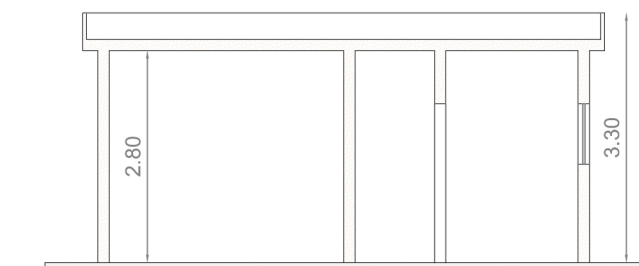
Sezione Y-Y'
