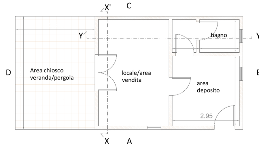
Pianta
