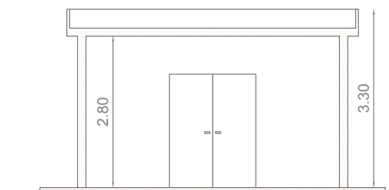
Sezione X-X'
