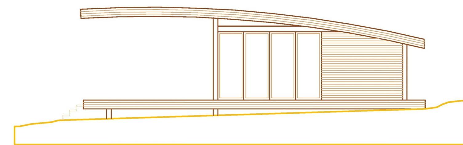
SEZIONE X-X
