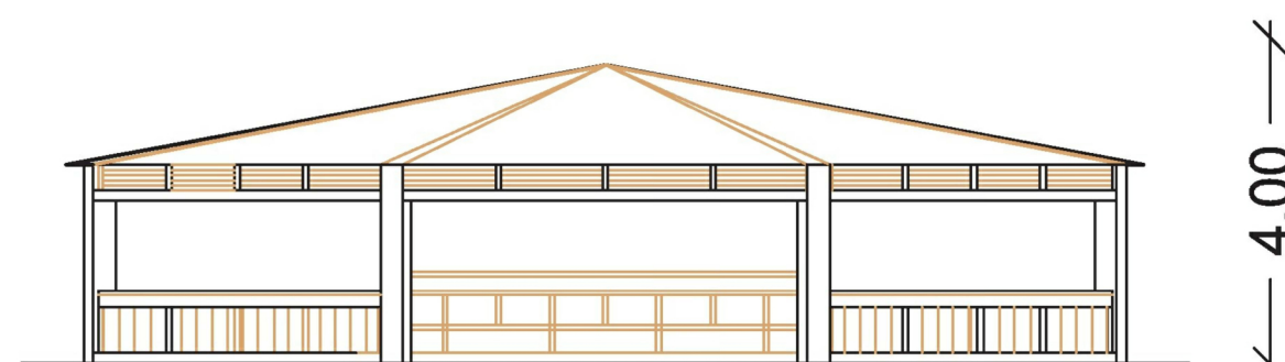
SEZIONE X-X
