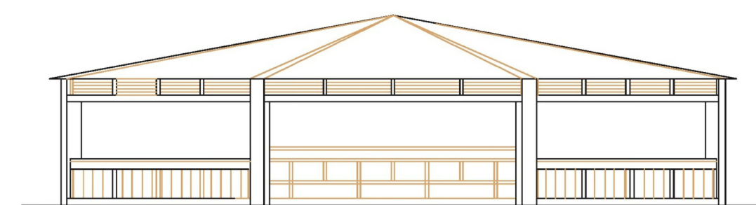
PROSPETTO POSTERIORE
