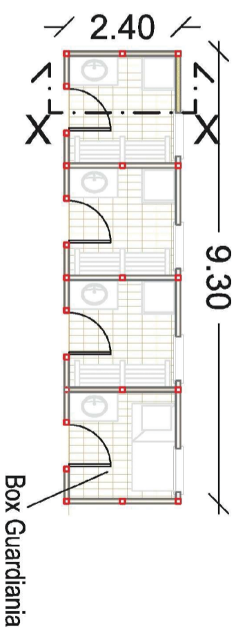
PIANTA SCHEMA TIPO INTERNO
